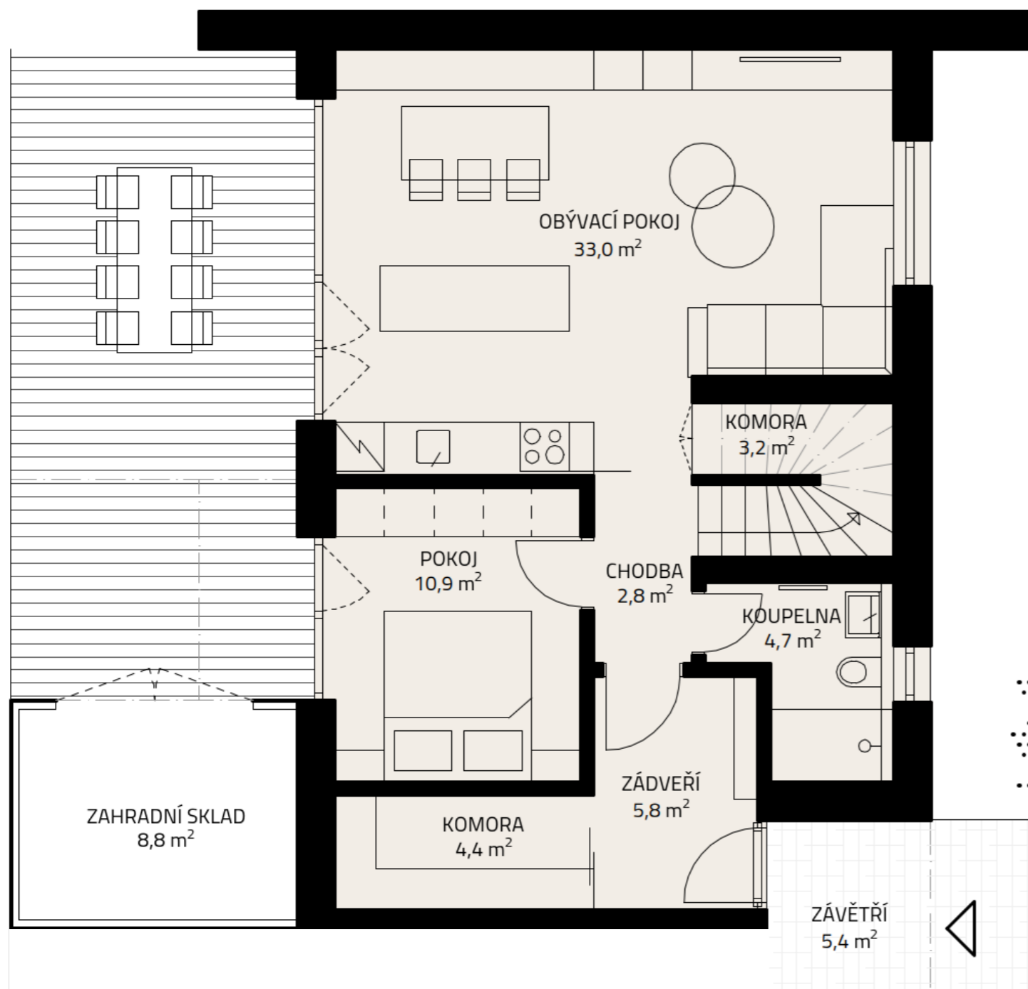
PŮDORYS PŘÍZEMÍ
