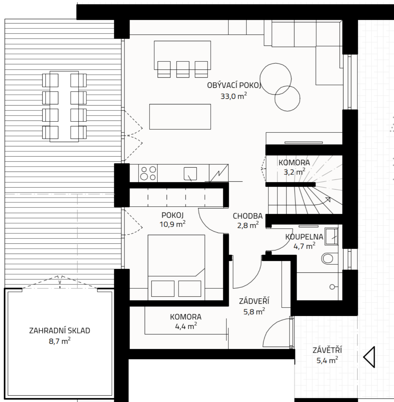
PŮDORYS PŘÍZEMÍ
