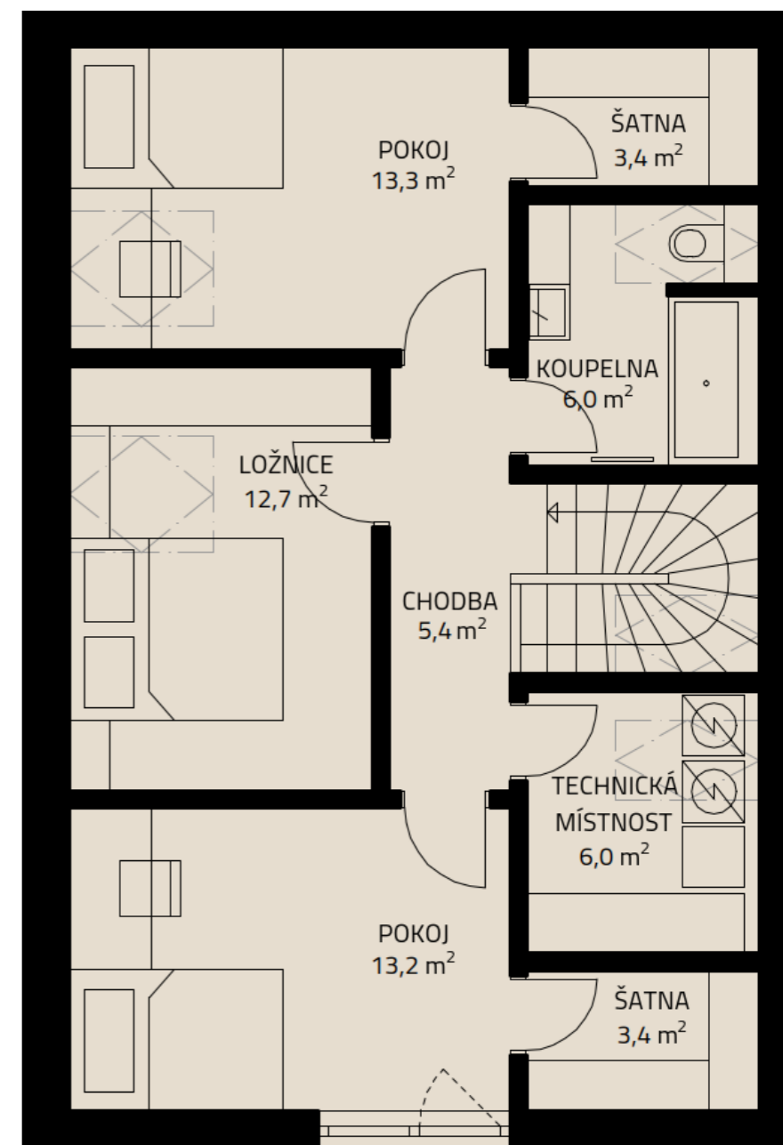
PŮDORYS PODKROVÍ
