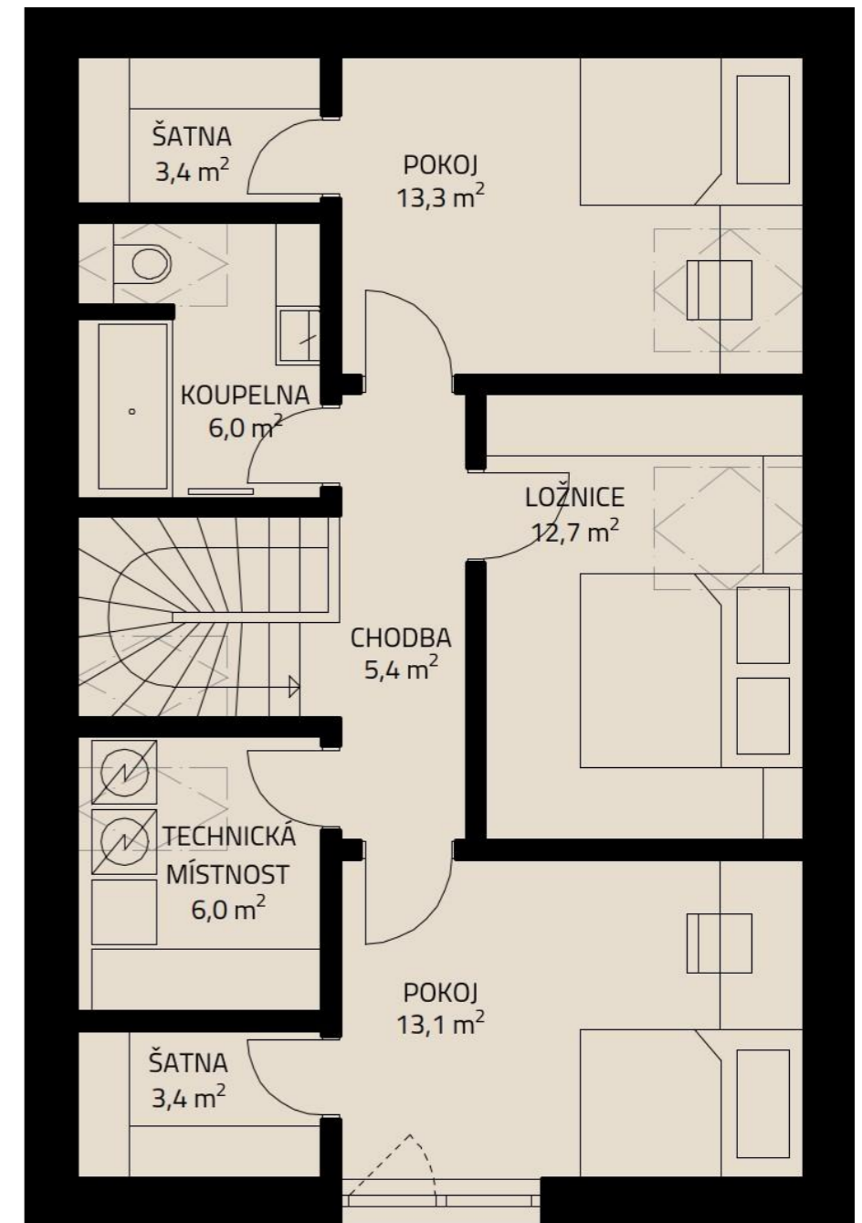
PŮDORYS PODKROVÍ
